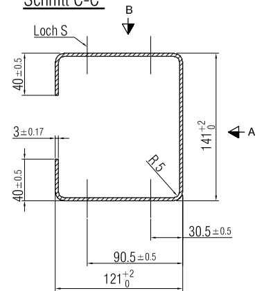
Schnitt C-C
