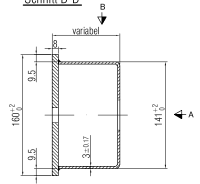
Schnitt D-D
