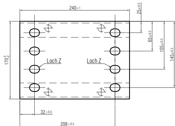
Ansicht A
