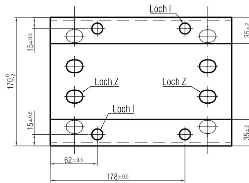
Ansicht B
