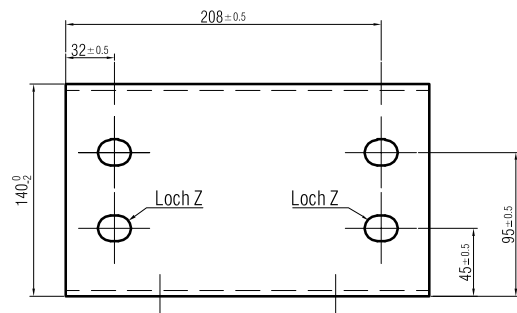
Ansicht A
