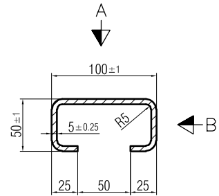
Querschnitt
