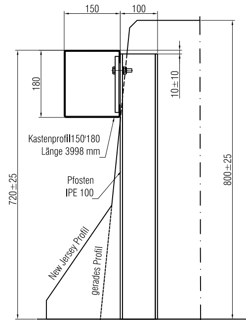
Schnitt B-B
