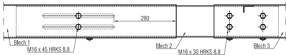
Draufsicht
