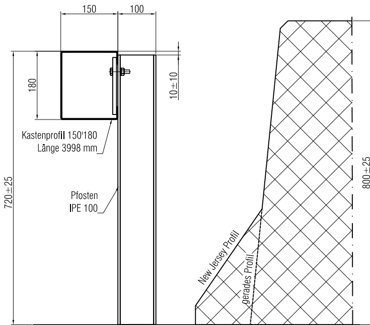
Schnitt B-B
