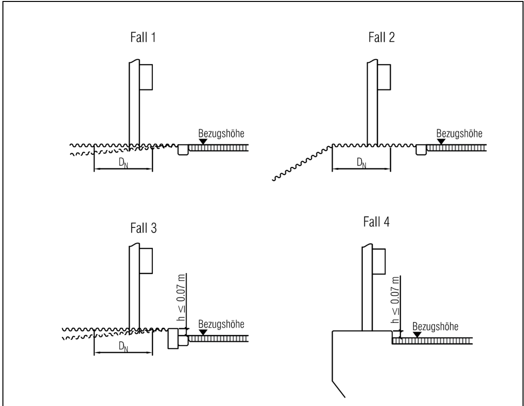
Abb. 6.1 Positionen und Bezugshöhen System 6211 (Anwendung, siehe Ziffer 6.2).
