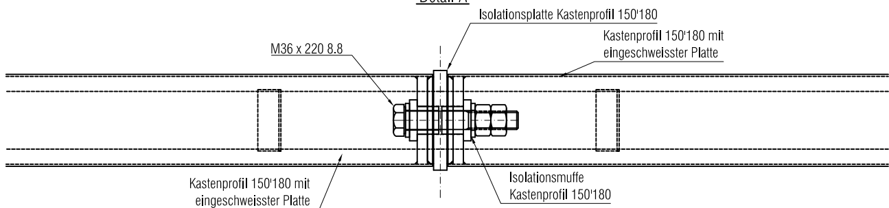
Draufsicht
