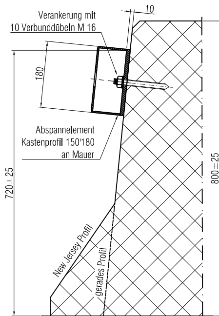
Schnitt A-A
