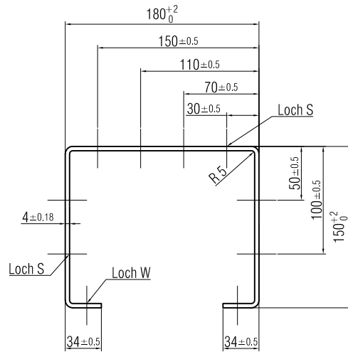
Ansicht von B
