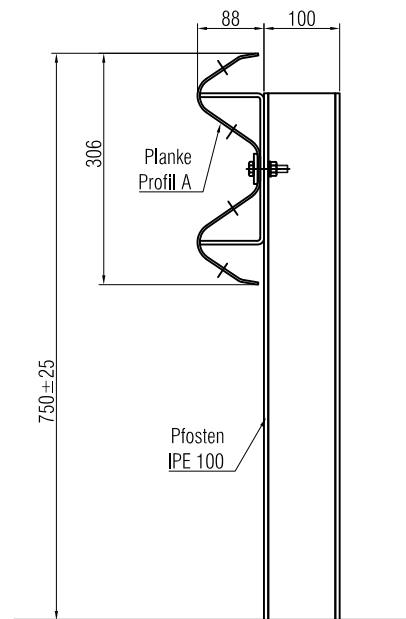
Schnitt A - A
