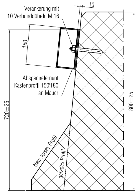
Schnitt A-A
