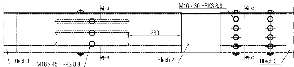
Draufsicht
