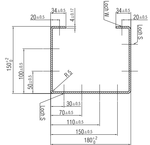
Schnitt C-C
