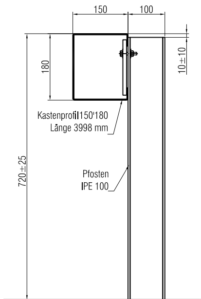
Schnitt B - B
